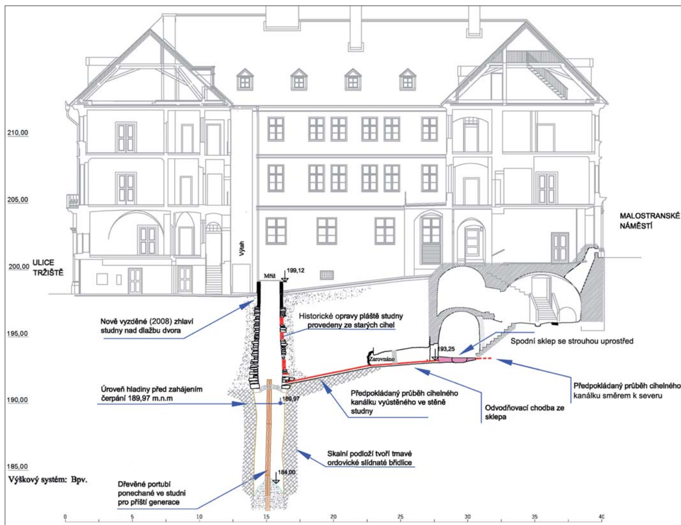
Obr. 16. Celkový řez odkrytou vodovodní a odvodňovací soustavou v domě „U tří zlatých korun“ (zaměření a zpracování SPELEO – Řehák a J. Hlavatý, 2009).
